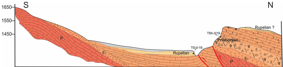
Նկար 2. Շաղափի սինկլինալի հարավային հատվածի կտրվածք: P- պերմի կրաքարեր, E1 – ստորին էոցենի կոնգլոմերատներ, օրգանածին կրաքարեր (Sahakyan et al., 2020).
