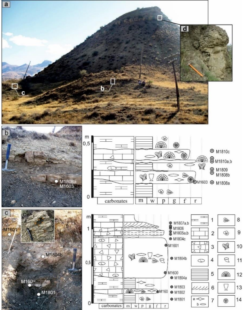
Նկար 3. Մալիշկա կտրվածքի դաշտային նկարը (Grigoryan et al., 2026): a - ընդհանուր տեսքը; b - c - Ուրցածորի շերտախմբի ստորին հատվածը, c' - կրաքարերում հանդիպող հրաբխային խճաքարեր (կետագծով նշված); d - Շաղափի շերտախմբի վերին հատվածի ավազաքարեր: 1 - մերգելներ, 2 - օրգանոգեն կրաքարեր, 3 - էքստրակլաստային կրաքարեր, 4 -կարբոնատային և բազալտային խիճ/խճաքարեր, 5 - զուգահեռ շերտավորում, 6 - խաչաձև շերտավորում (թույլ արտահայտված կառուցվածքները նշված են կետագծով):
